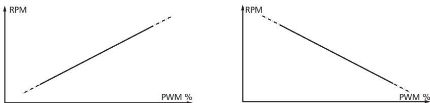
Fig. 6 : Caractéristiques des pompes à haute efficacité avec profil PWM d'une courbe croissante (AA, gauche) et décroissante (Ab, droite)
