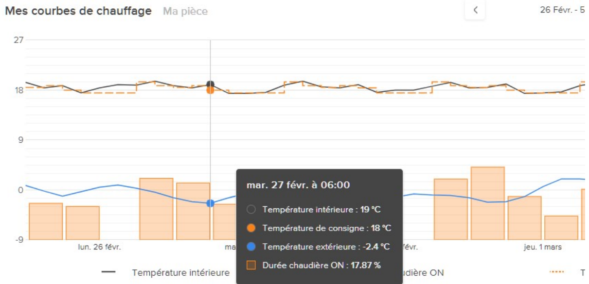
Figure 9 Courbe de chauffage au plus froid de l'hiver 2018
